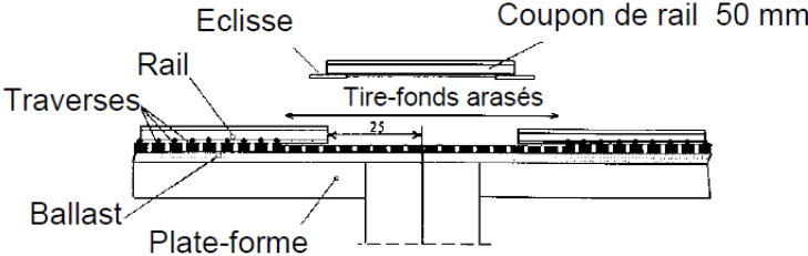
Figure 3 Assemblage de deux modules.
